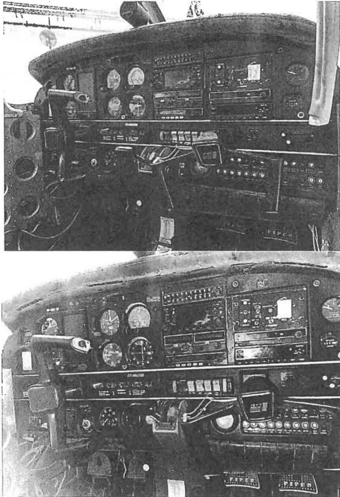
Ilustración 6. Panel de Instrumentos
