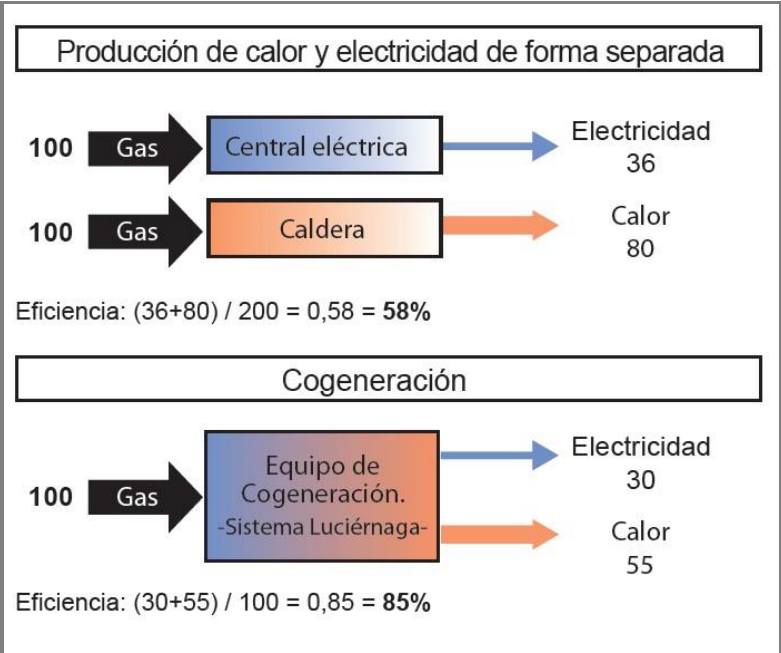
FIGURA 76- Producción de calor y electricidad de forma separada vs. Cogeneración
