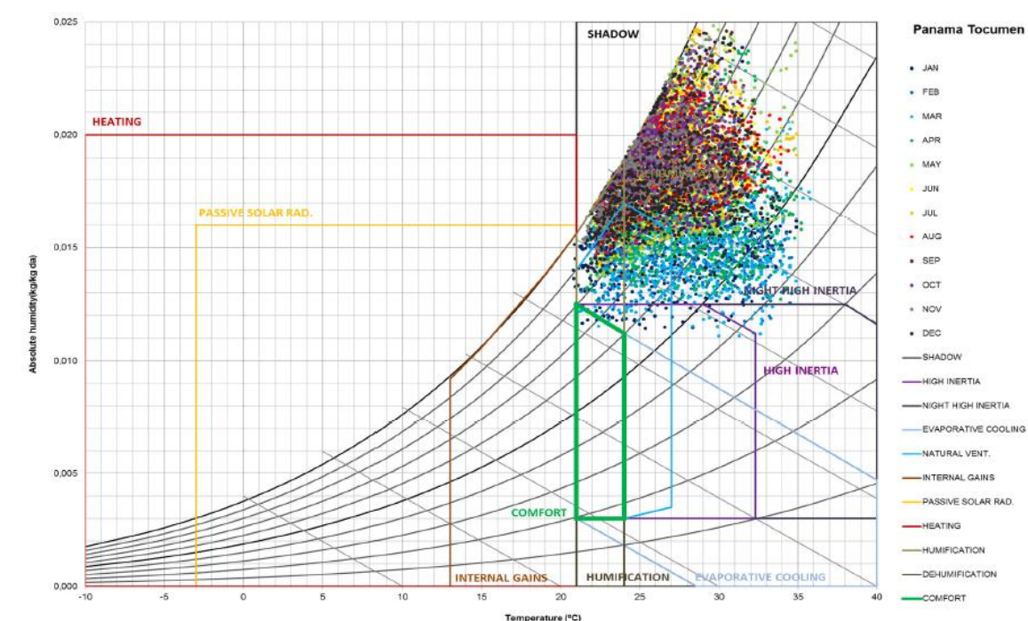
• Gráfico de Givoni y las principales estrategias bioclimáticas (Datos de la estación Aeropuerto Tocumen WMO 787920 Panamá)
