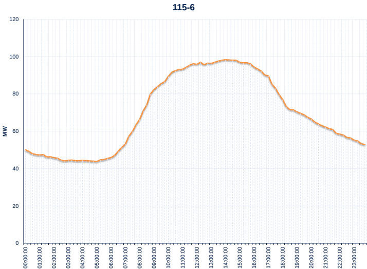
Gráfico 33: Curva Típica de Carga Línea 115-6
