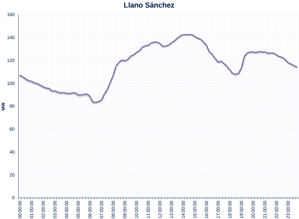
Gráfico 39: Curva Típica de Carga Llano Sánchez
