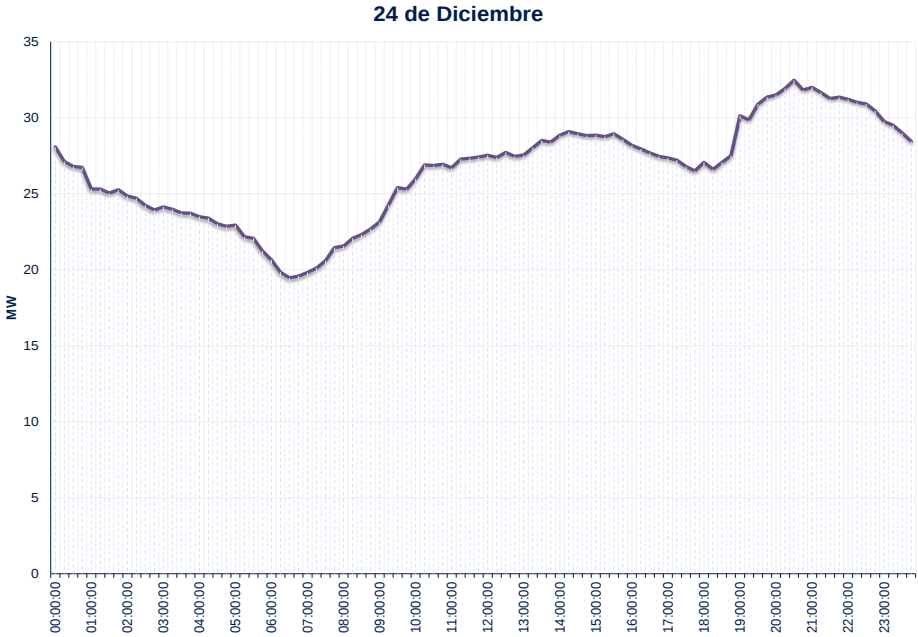
Gráfico 53: Curva Típica de Carga 24 de Diciembre
