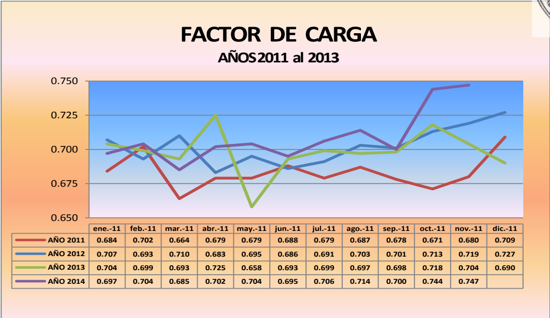
Gráfico 19: Factor de Carga
