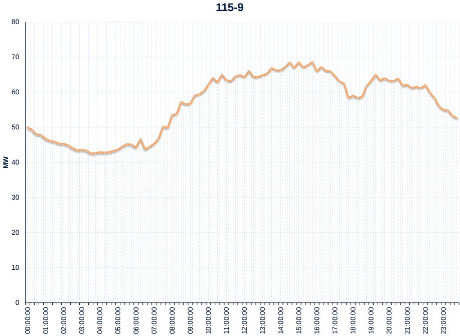
Gráfico 47: Curva Típica De Carga Línea 115-9
