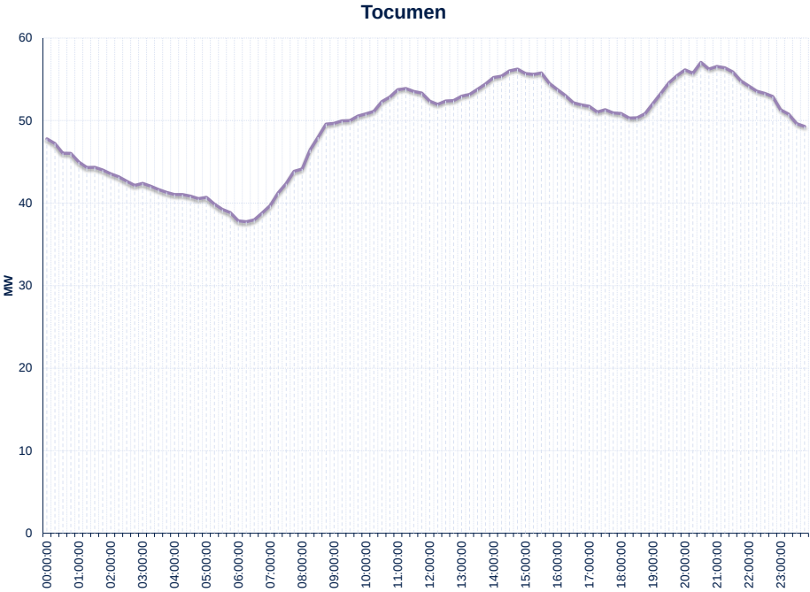
Gráfico 45: Curva Típica De Carga Tocumen
