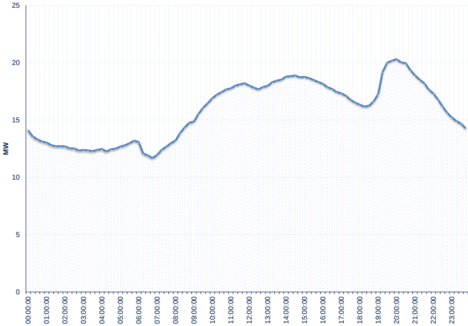
Gráfico 41: Curva Típica De Carga Progreso
