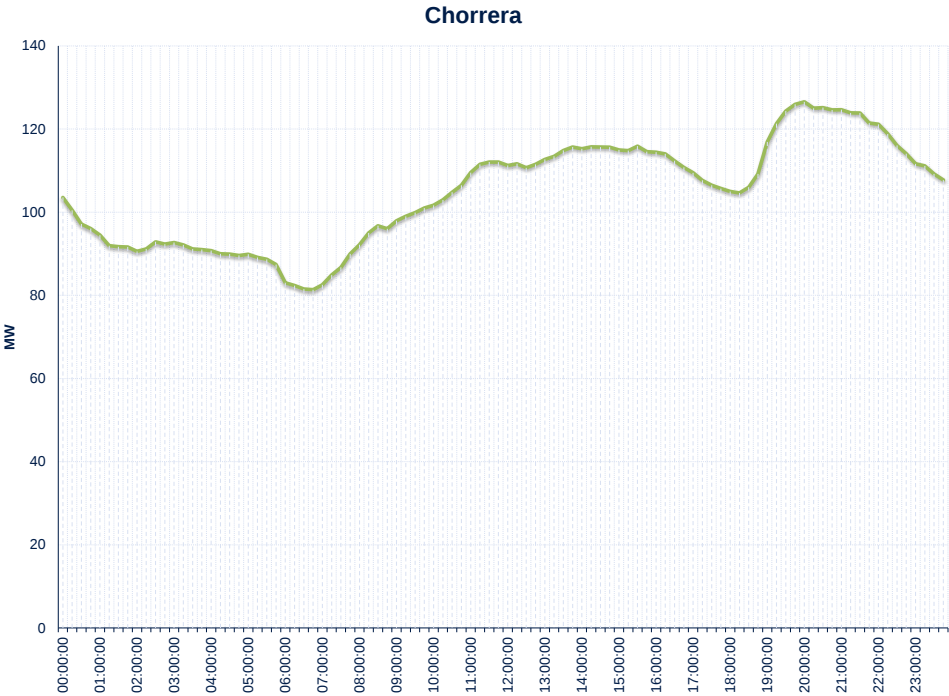
Gráfico 38: Curva Típica De Carga Chorrera
