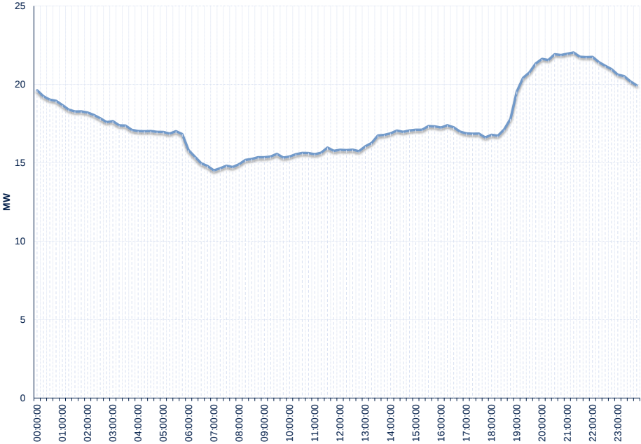
Gráfico 42: Curva Típica De Carga Las Minas 44
