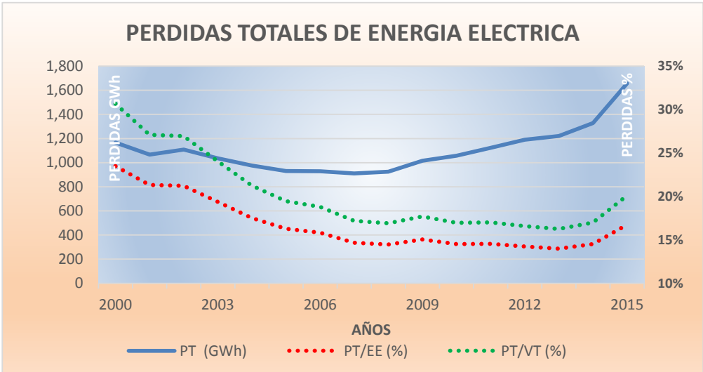
Gráfico 21: Pérdidas Totales de Energía Eléctrica
