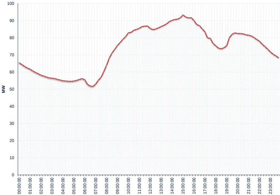
Gráfico 40: Curva Típica De Carga Mata de Nance
