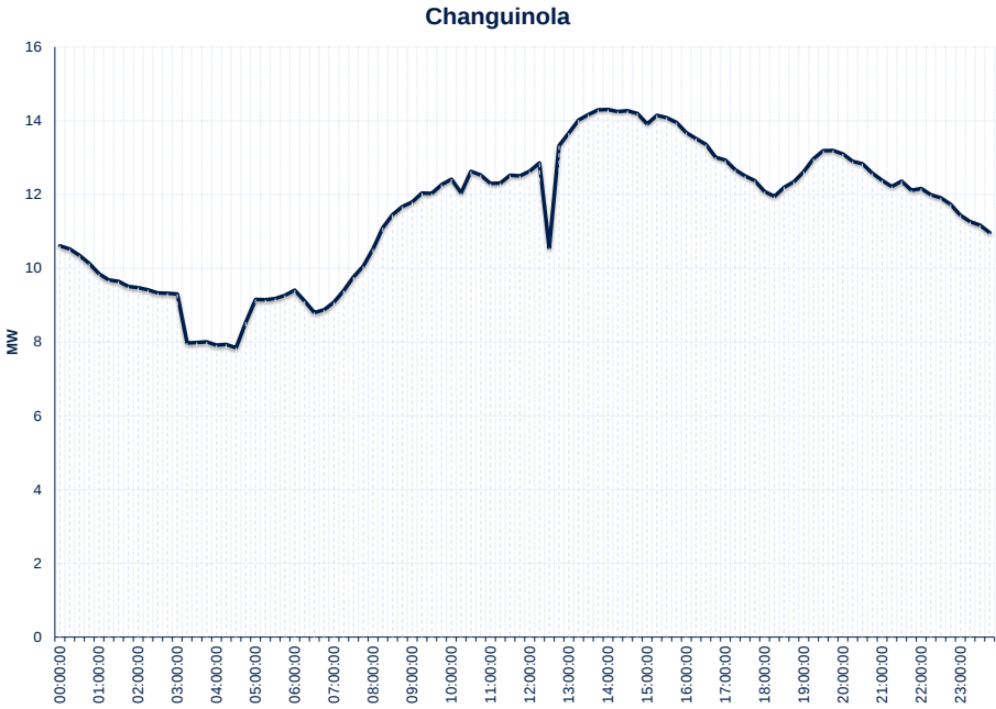
Gráfico 55: Curva Típica De Carga Changuinola
