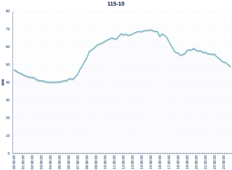
Gráfico 46: Curva Típica De Carga Línea 115-10
