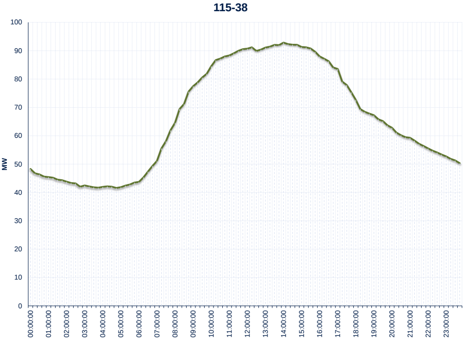
Gráfico 36: Curva Típica de Carga Línea 115-38
