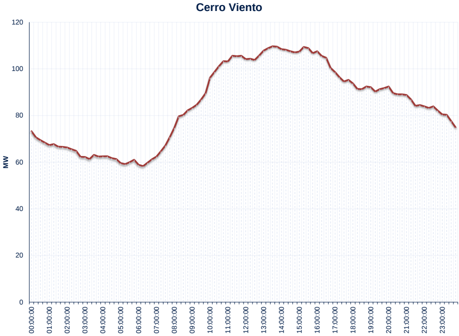
Gráfico 49: Curva Típica de Carga Cerro Viento
