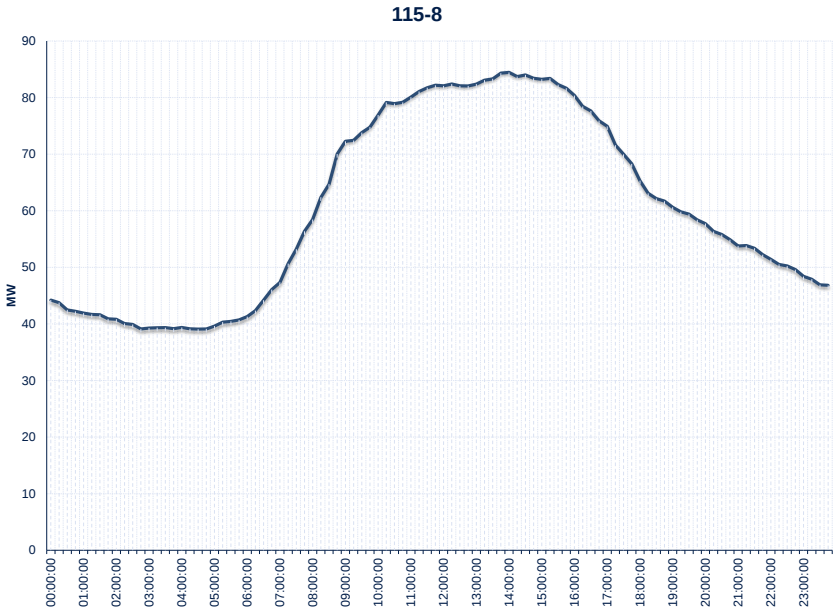
Gráfico 34: Curva Típica de Carga Línea 115-8
