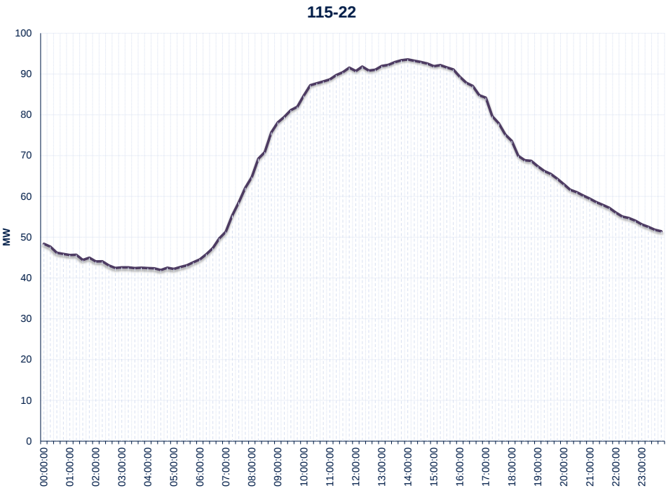
Gráfico 37: Curva Típica de Carga Línea 115-22
