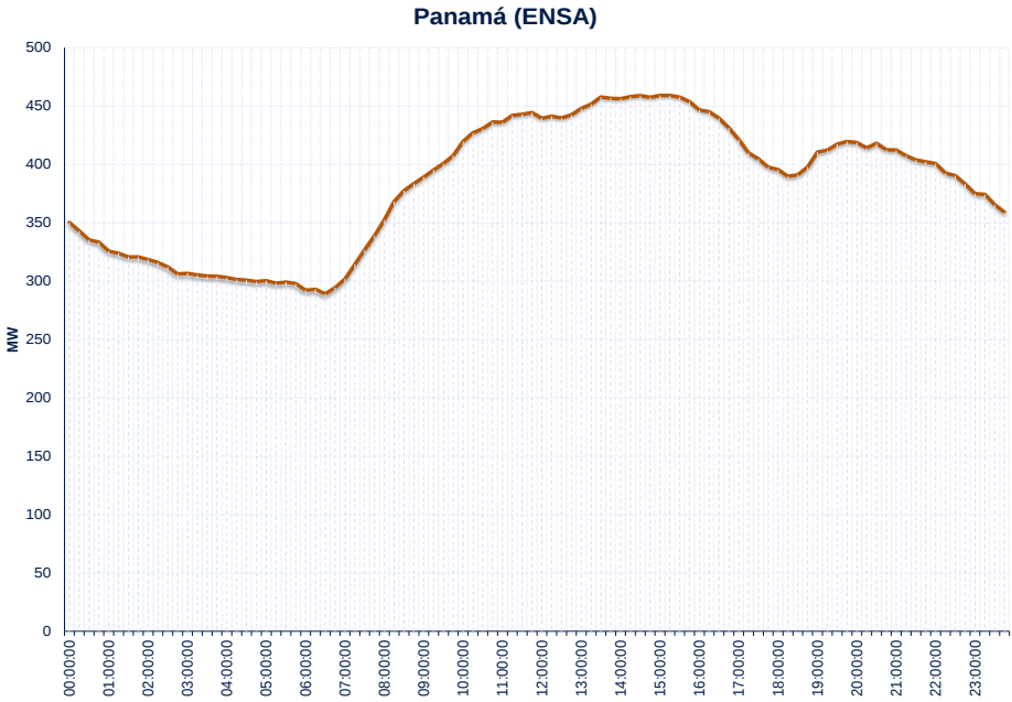
Gráfico 52: Curva Típica de Carga ENSA – Panamá (Provincia de Panamá - S/E Panamá, S/E Cerro Viento, S/E Geehan, S/E Tocumen, S/E Santa María y S/E 24 De Diciembre)
