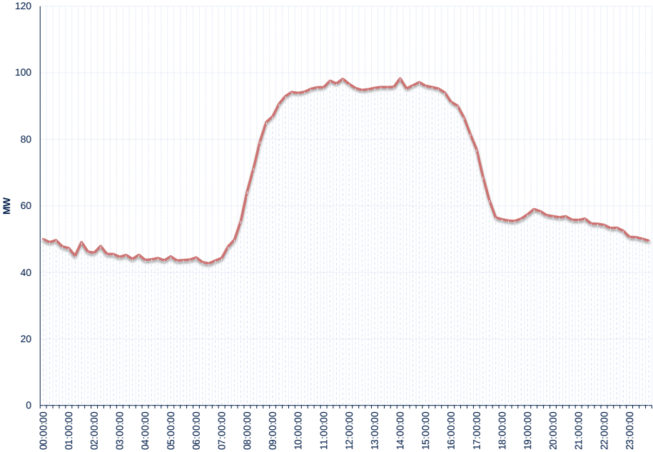
Gráfico 43: Curva Típica De Carga France Field 115
