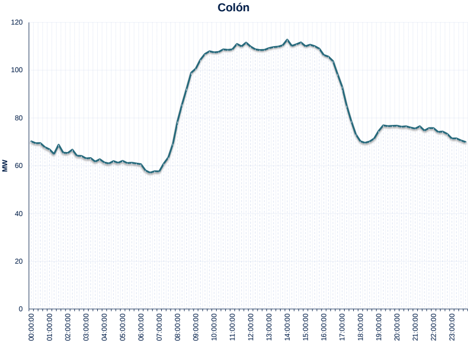
Gráfico 51: Curva Típica de Carga Provincia de Colón (S/E France Field, S/E BLM, S/E Colón 1 y S/E Monte Esperanza)
