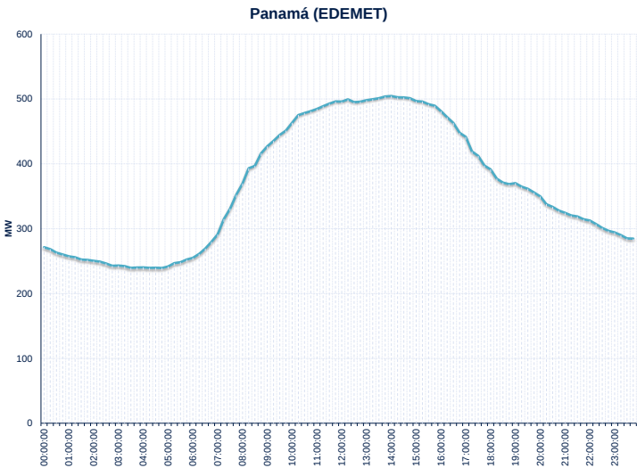
Gráfico 32: Curva Típica de Carga EDEMET – Panamá
