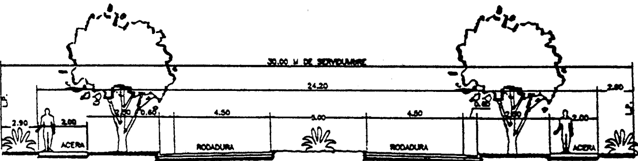
SECCION CARACTERISTICA DE VIA SECUNDARIA EN AREA INDUSTRIAL
