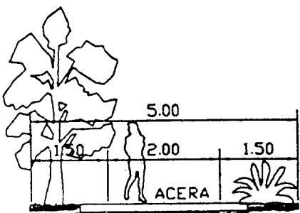
SERVIDUMBRE MINIMA DE VEREDA INDUSTRIAL, INSTITUCIONAL
