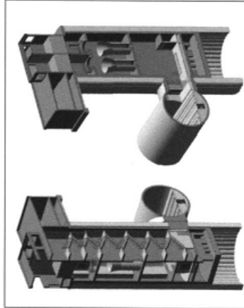
Fig. 10 – Sección Constructiva Pozo Ventilación y Salida Emergencia
